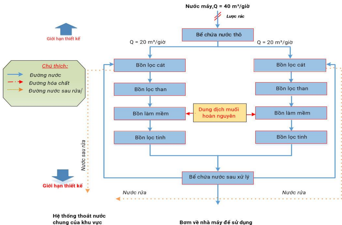
Sơ đồ quy trình xử lý nước cấp
